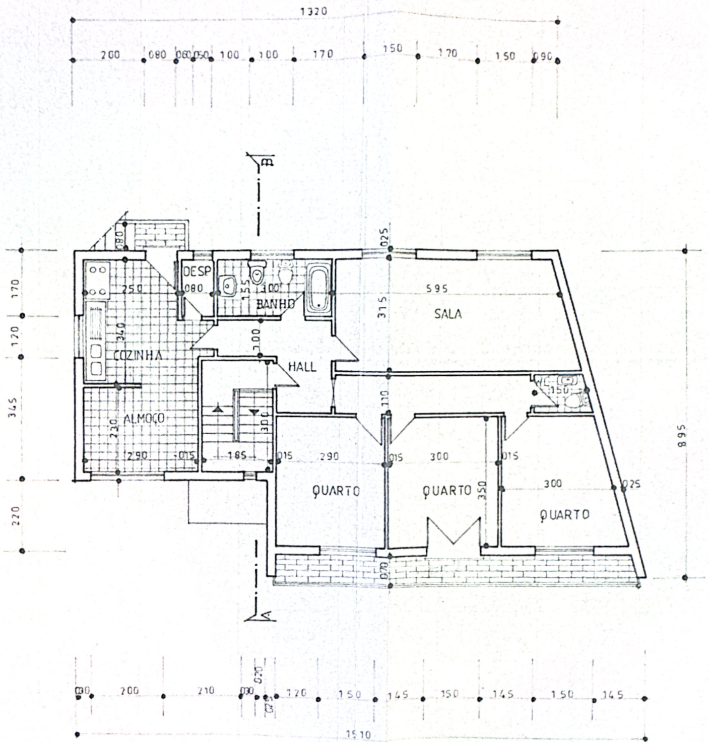
PLANTA DO 2º PISO
